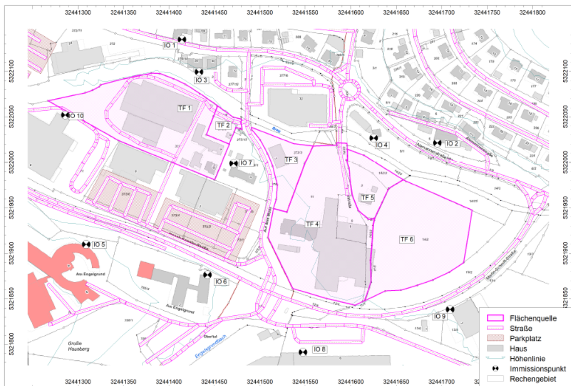
Computermodell mit Immissionsorten u. Flächenschallquellen für Teilflächen (Quelle: GN Bauphysik; o. M.)
